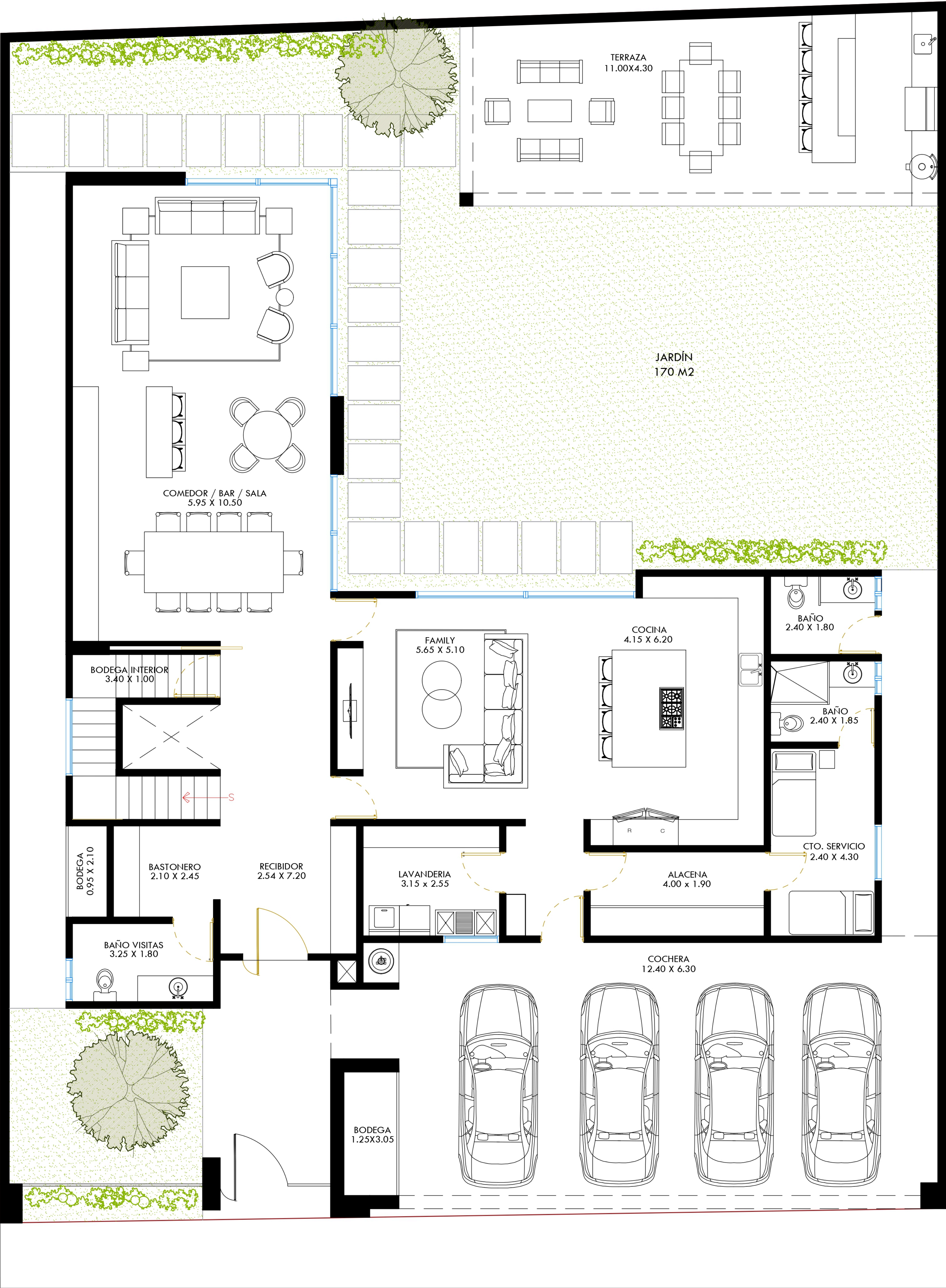
PLANTA BAJA
