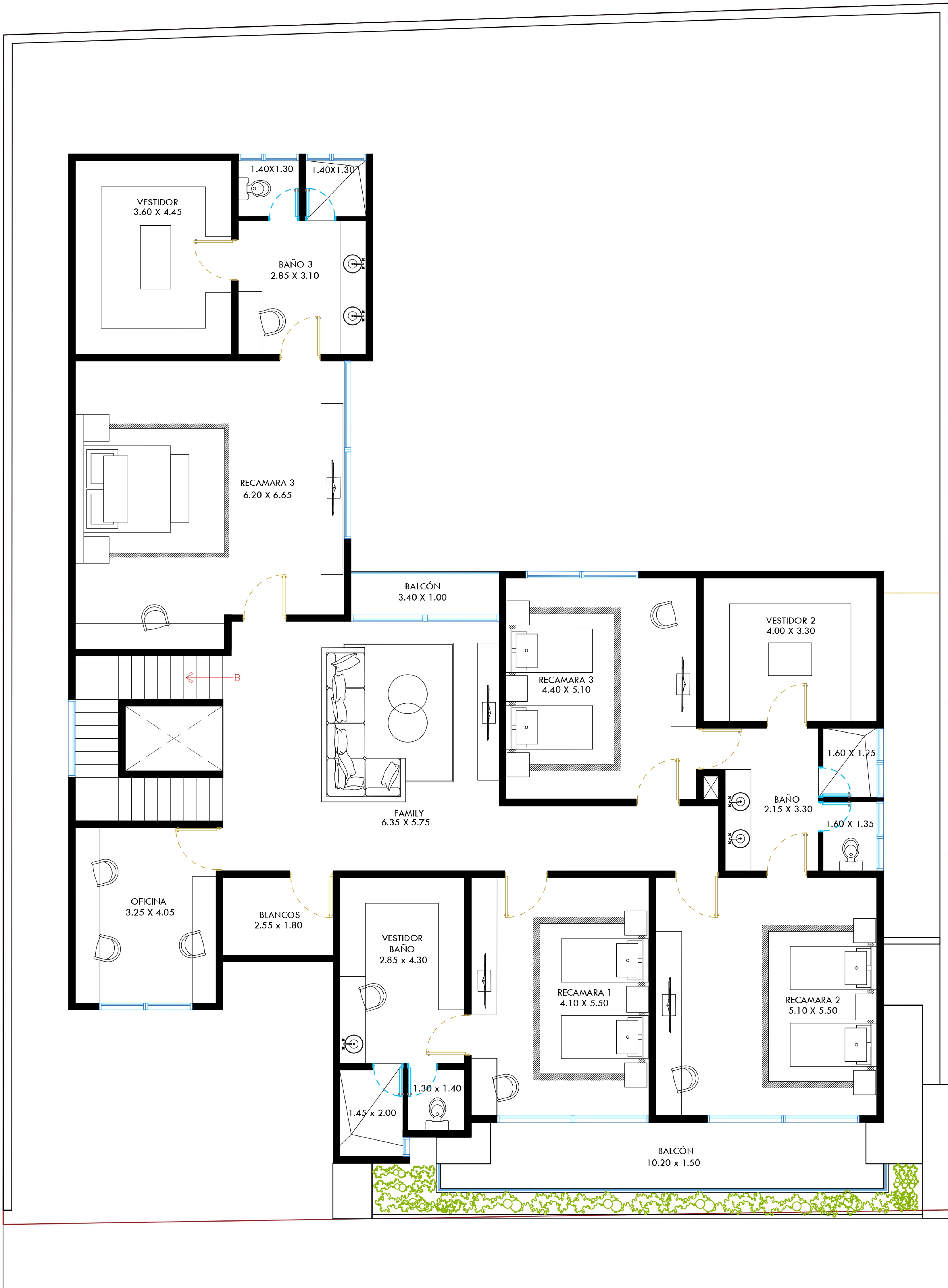
PLANTA ALTA
